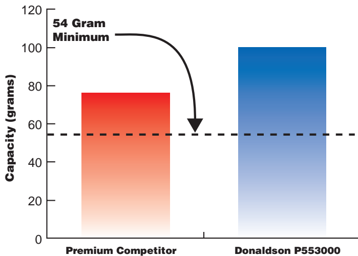
Capacity Per SAE J1858
