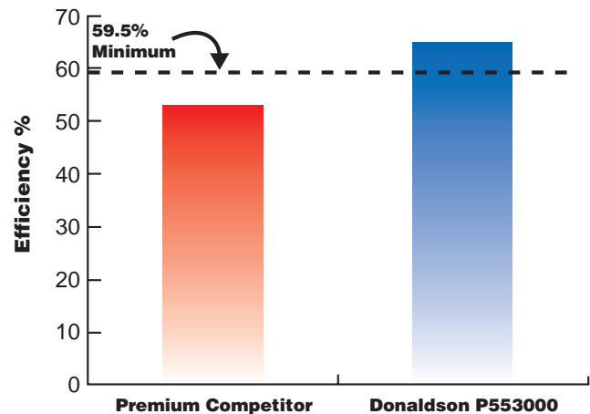
Efficiency Per SAE J1858
